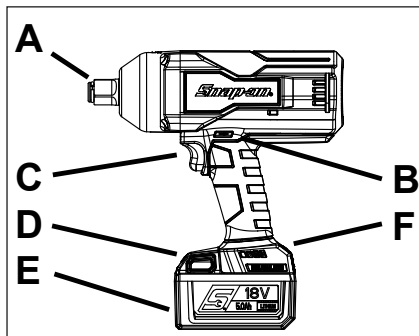
図 1: コードレスインパクトレンチ
