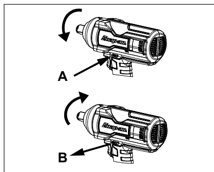
Figure 3: Commutatore del senso di rotazione
