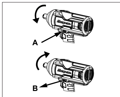
Figura 3: Interruptor de avance / marcha atrás
