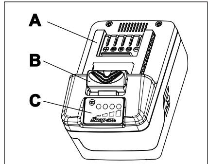
Abbildung 7: Akku (CTB8187)
