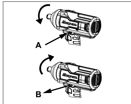
Figure 3 : Commutateur avant/arrière
