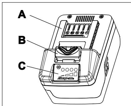
図 7: バッテリーパック (CTB8187)
